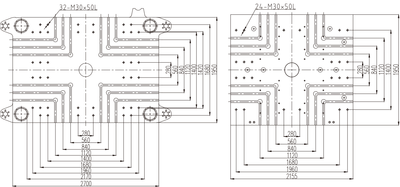
上模板/Upper Plate
