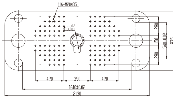
上模板/Upper Plate
