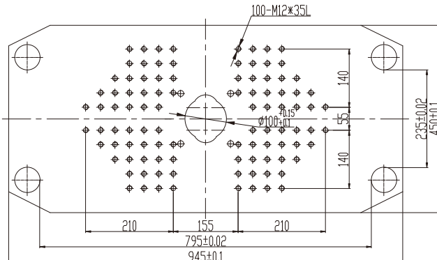
上模板/Upper Plate
