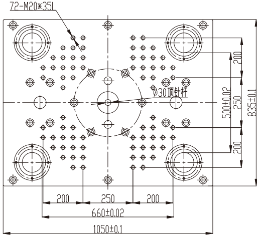
下模板/Below Plate
