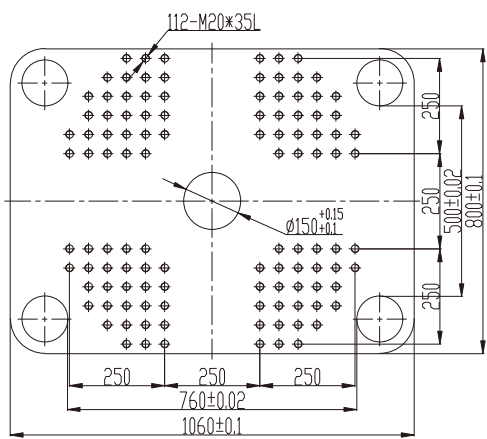
上模板/Upper Plate
