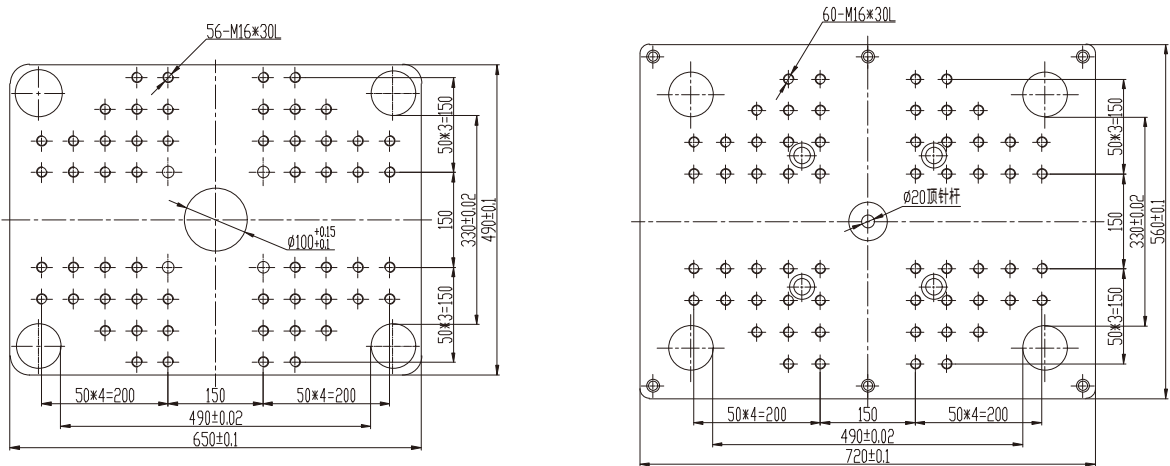
上模板/Upper Plate
