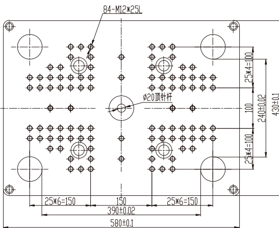
下模板/Below Plate
