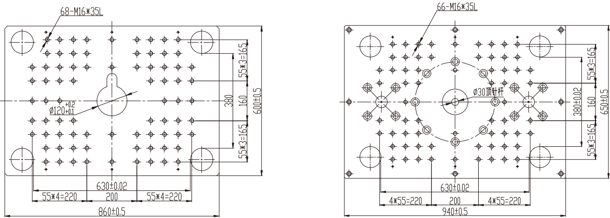
上模板/Upper Plate
