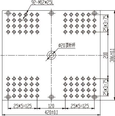
单滑板/Single Slide
