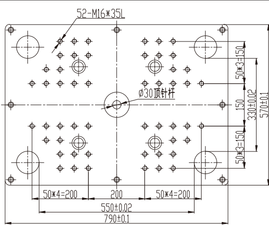
下模板/Below Plate
