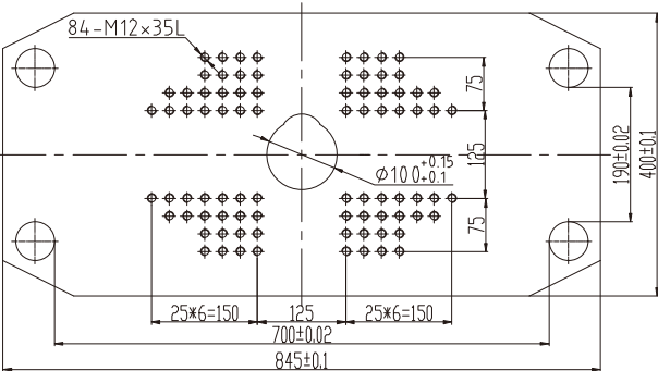
上模板/Upper Plate
