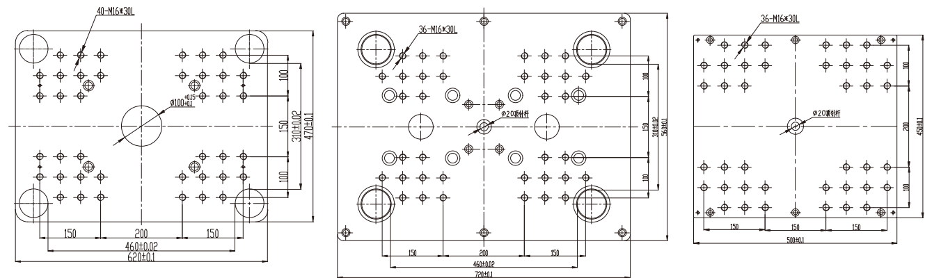
上模板/Upper Plate
