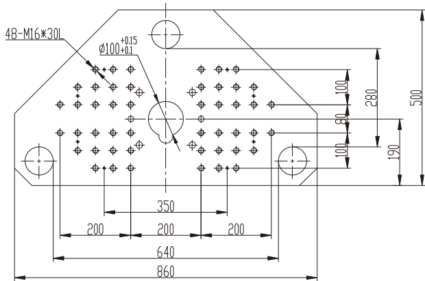
上模板/Upper Plate
