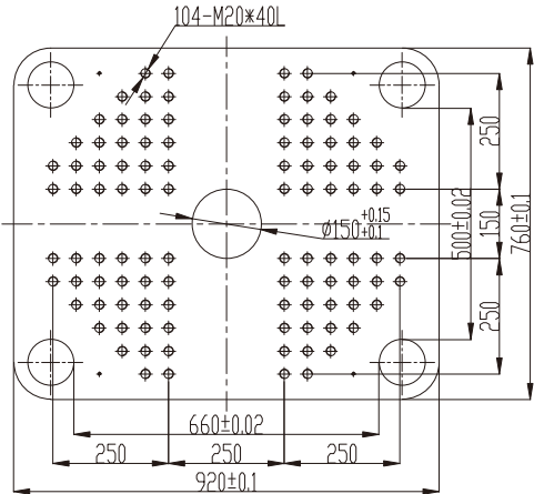
上模板/Upper Plate
