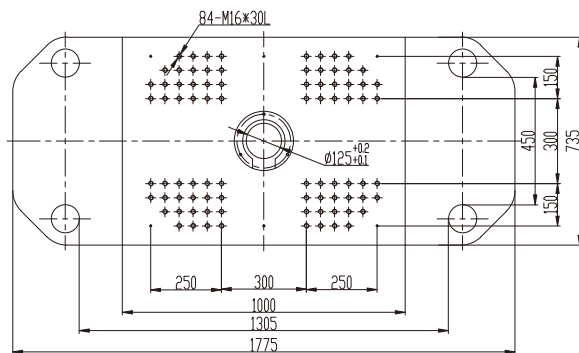
上模板/Upper Plate
