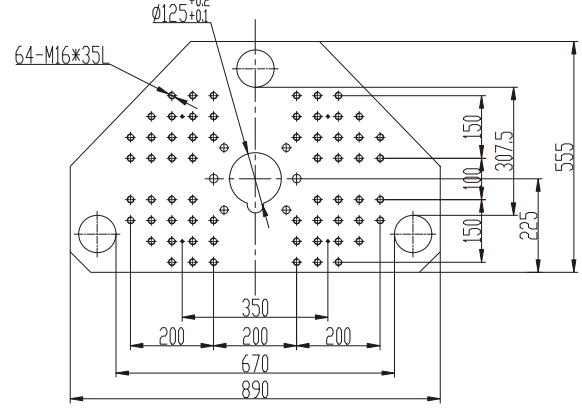
上模板/Upper Plate
