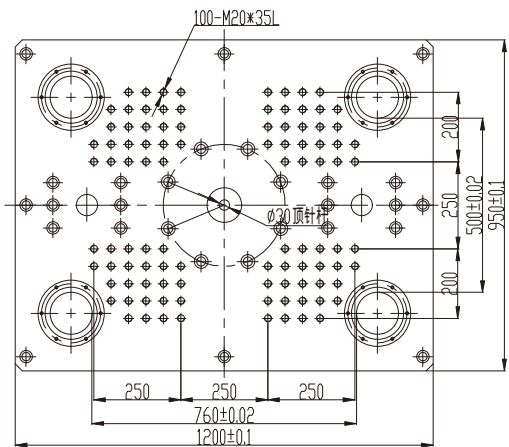
下模板/Below Plate
