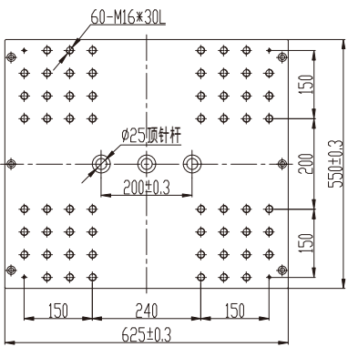
单滑板/Single Slide
