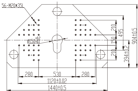
上模板/Upper Plate
