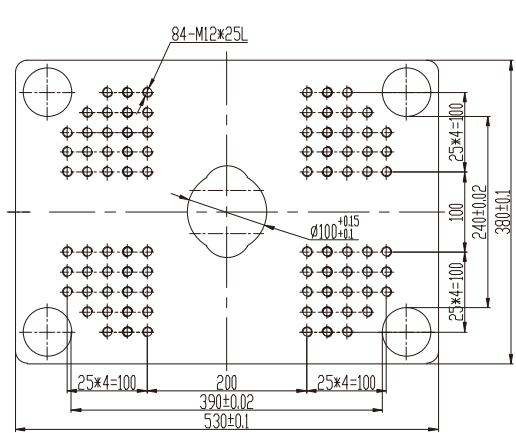
上模板/Upper Plate
