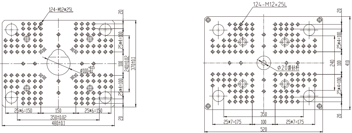
上模板/Upper Plate
