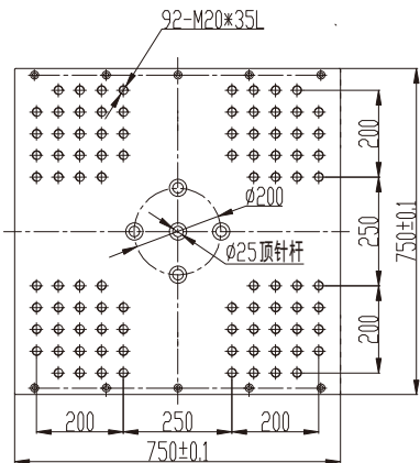
下滑板/Below Slide
