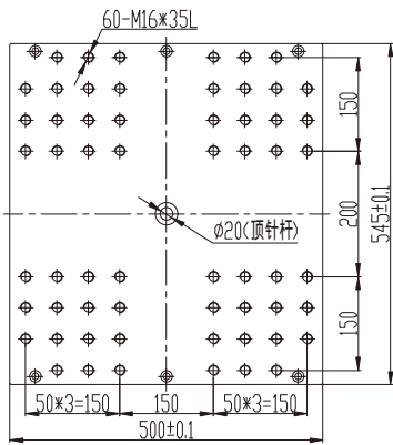
单滑板/Single Slide
