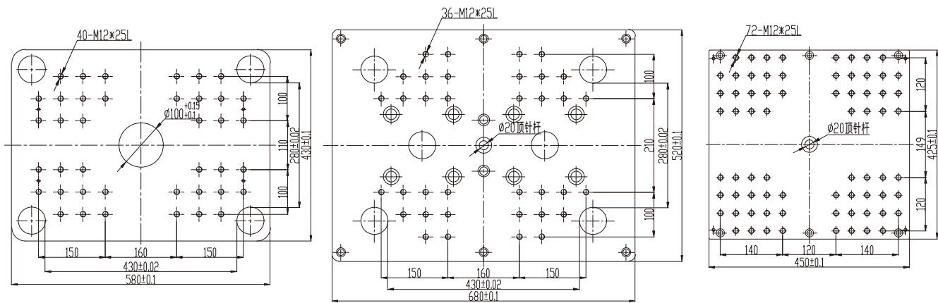
上模板/Upper Plate
