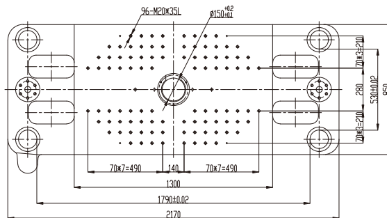
上模板/Upper Plate
