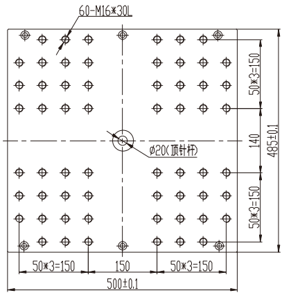
单滑板/Single Slide
